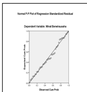
Gambar 2. Grafik Plot (P-Plot)
