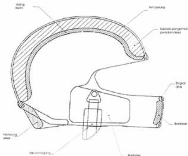
Gambar 1 Contoh konstruksi dan bagian-bagian helm standar tertutup ( full face ) (sumber: Badan Standarisasi Nasional www.bsn.go.id tahun 2009)
