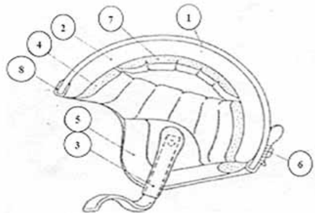
Gambar 2 Contoh konstruksi dan bagian-bagian helm standar terbuka ( open face ) (sumber: Badan Standarisasi Nasional www.bsn.go.id tahun 2009)
