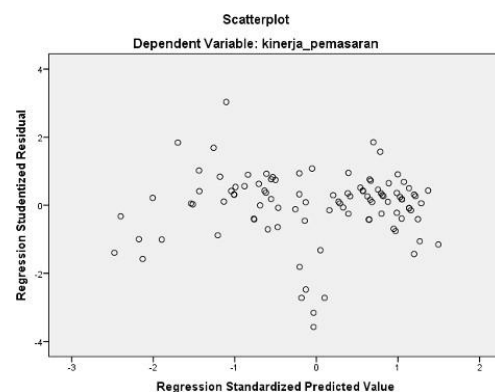
Gambar 1. Uji Heteroskedastisitas
