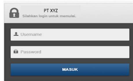
Gambar 4. Tampilan Login
